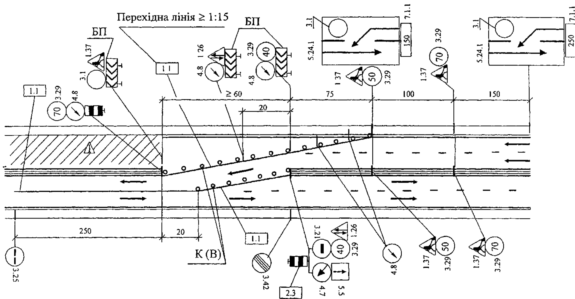
Схема А.28 ОДР в місцях початку виконання робіт при реконструкції та капітальному ремонті доріг I категорії
