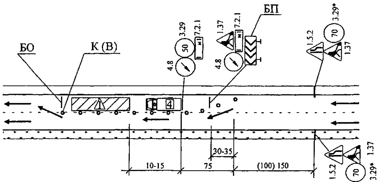
Схема А.8 Нанесення розмітки по трафаретах або лекалах на правій смузі дороги I категорії з чотирма смугами руху
