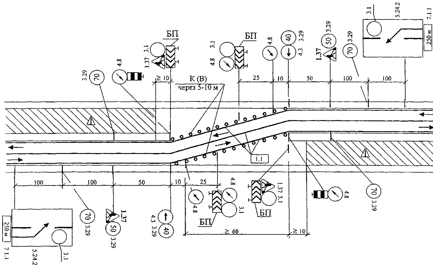
Схема А.30 ОДР в місцях переходу через розділювальну смугу справа наліво при реконструкції та капітальному ремонті доріг I категорії
