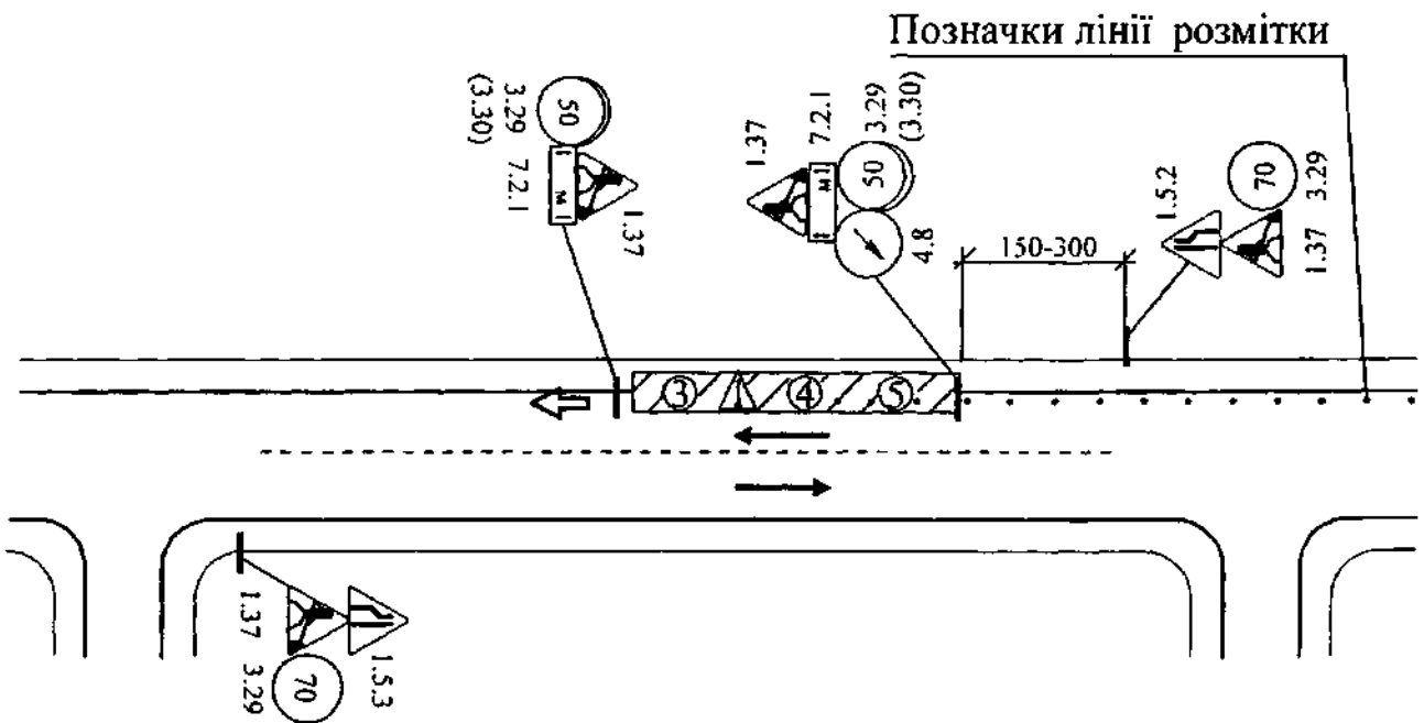
Схема А.2 Нанесення позначок лінії крайової розмітки вручну
