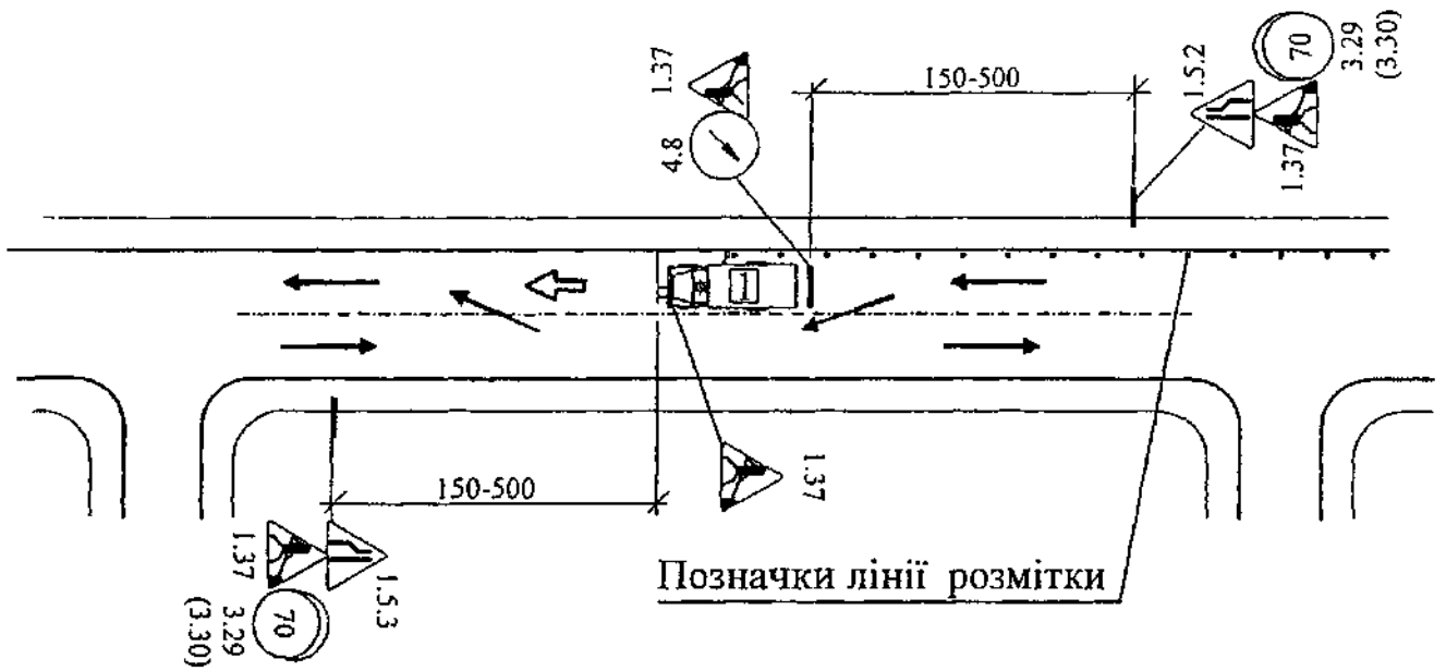
Схема А.3 Нанесення позначок лінії крайової розмітки автомобілем
