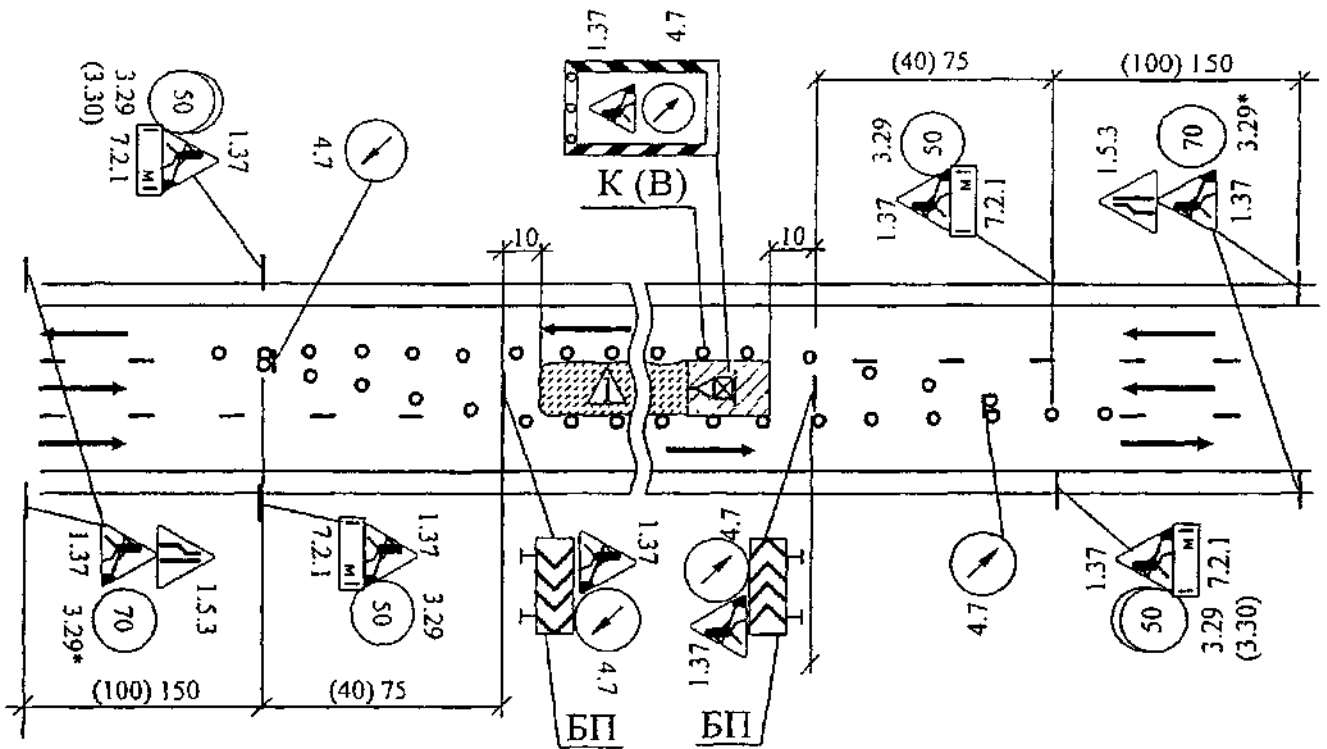
Схема А.23 ОДР при ремонті ділянок доріг з трьома смугами руху, виконанні натурних випробувань та досліджень покриття (8.8)
