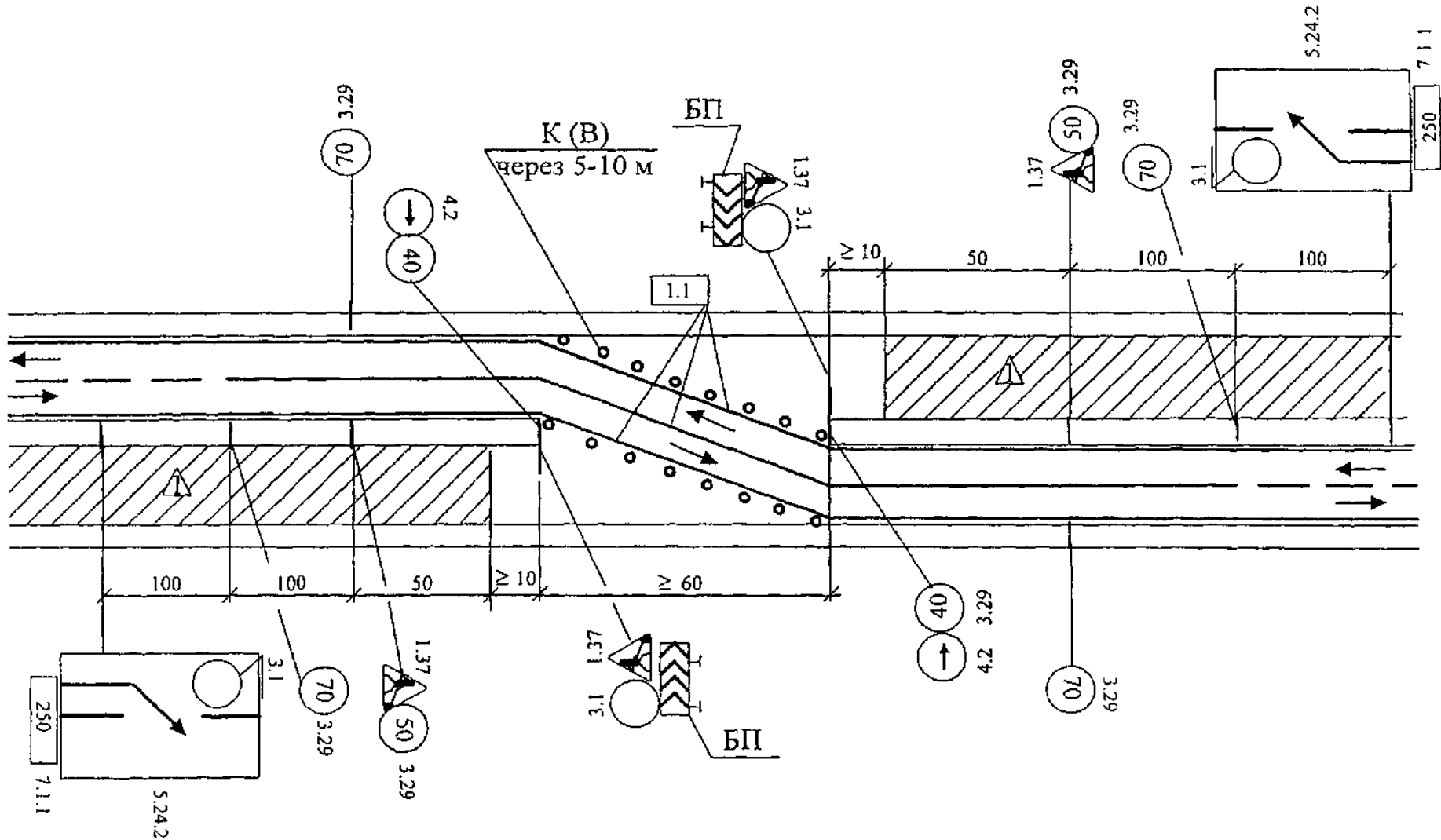
Схема А.29 ОДР в місцях переходу через розділювальну смугу зліва направо при реконструкції та капітальному ремонті доріг I категорії
