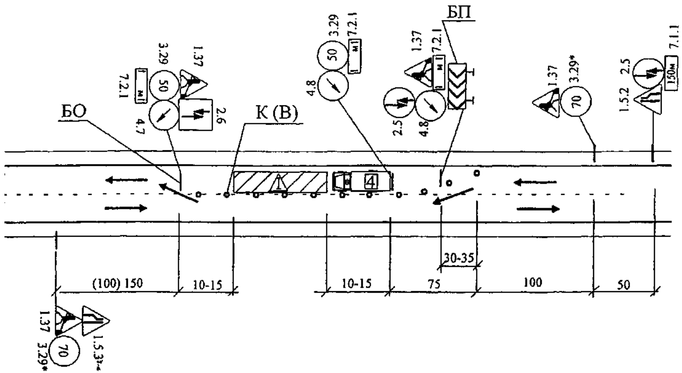
Схема А.7 Нанесення розмітки по трафаретах або лекалах на 2-х смугових дорогах за допомогою ручної розміточної машини
