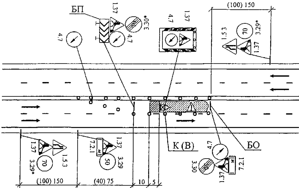
Схема А.25 ОДР при утриманні та ремонті внутрішньої смуги руху ділянок доріг з чотирма смугами руху, виконанні натурних випробувань та досліджень покриття (8,8)
