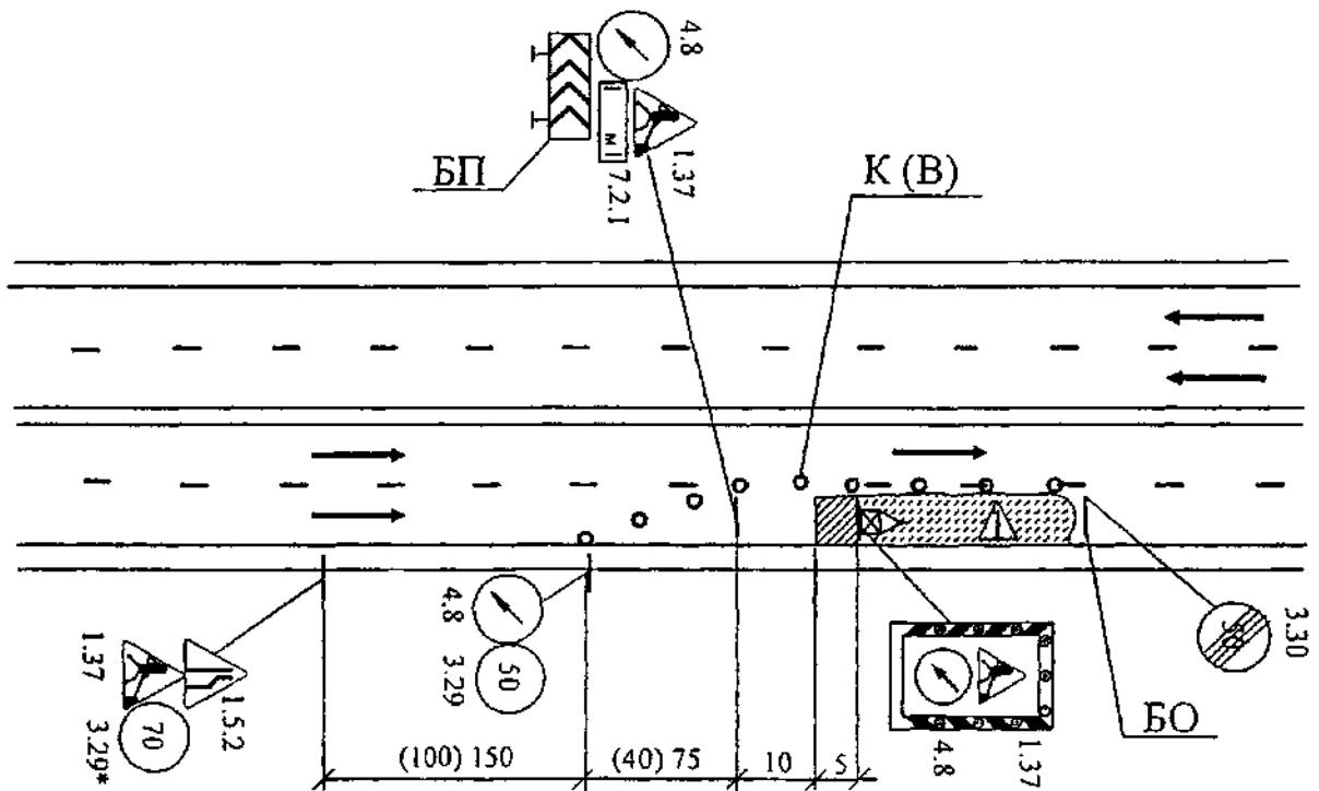
Схема А.23 ОДР при ремонті ділянок доріг з трьома смугами руху, виконанні натурних випробувань та досліджень покриття (8.8)
