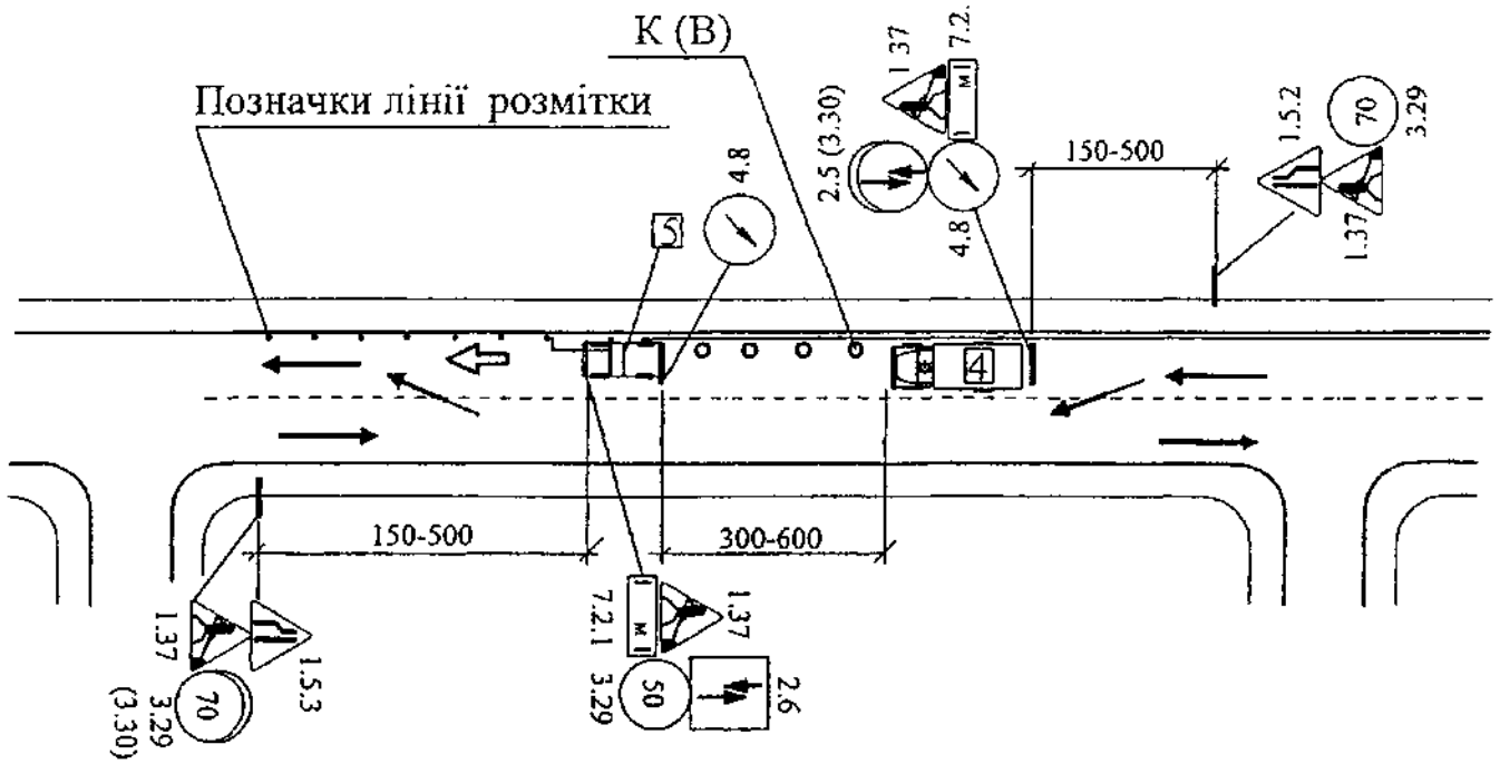
Схема А.5 Нанесення крайової лінії самохідною машиною
