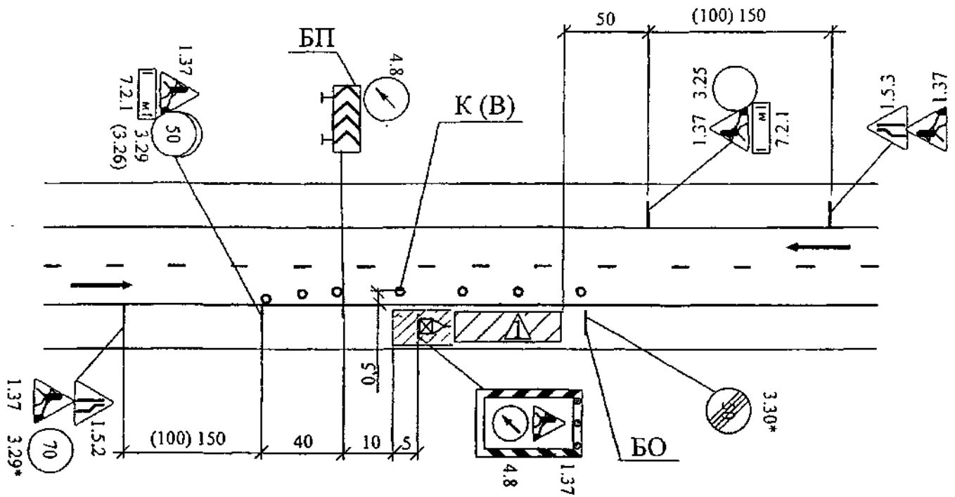
Схема А.15 ОДР при нанесенні вертикальної розмітки та поточному ремонті узбіччя, тротуару тощо
