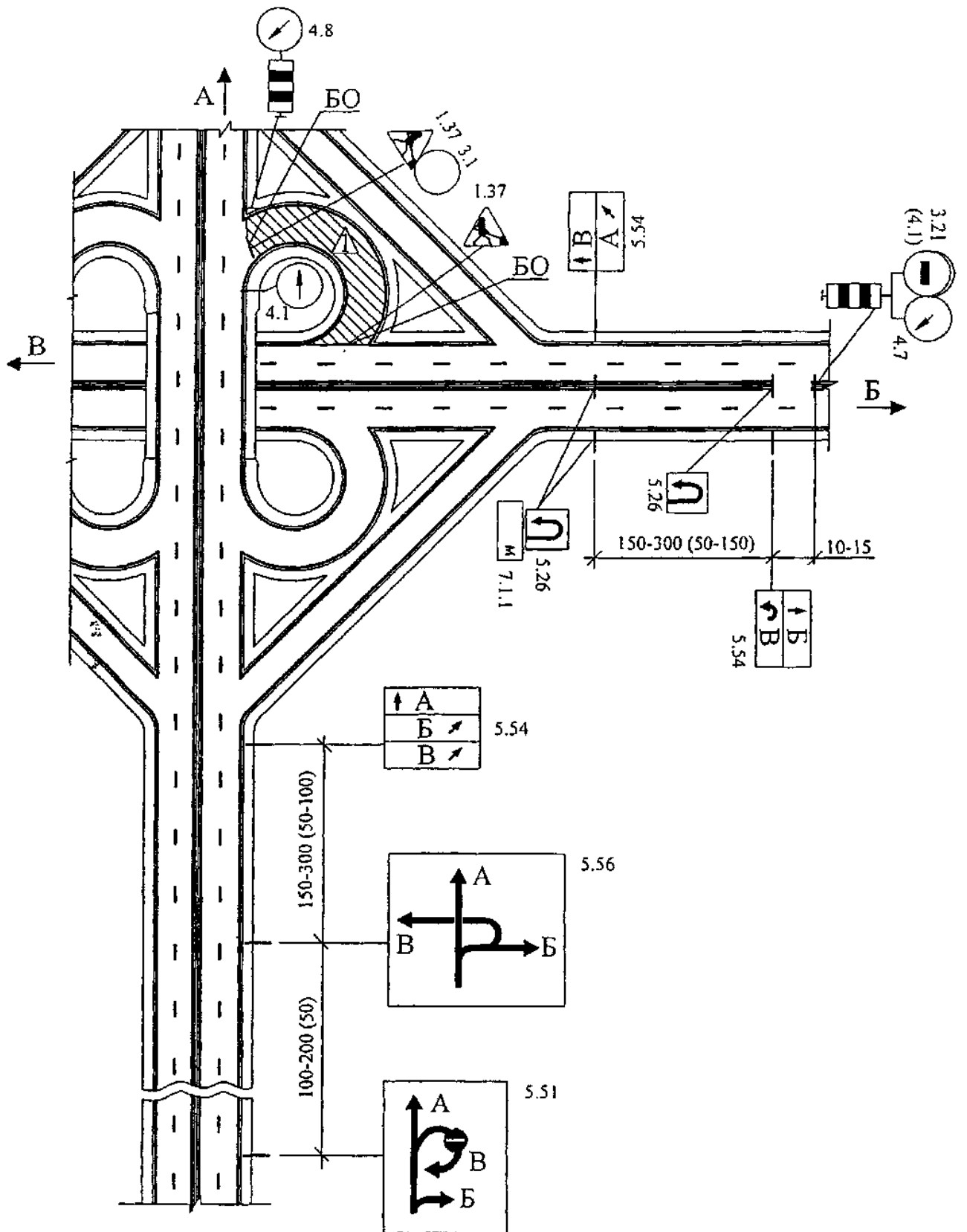
Схема А.27 ОДР при ремонті з'їзду на дорожній розв'язці у різних рівнях
