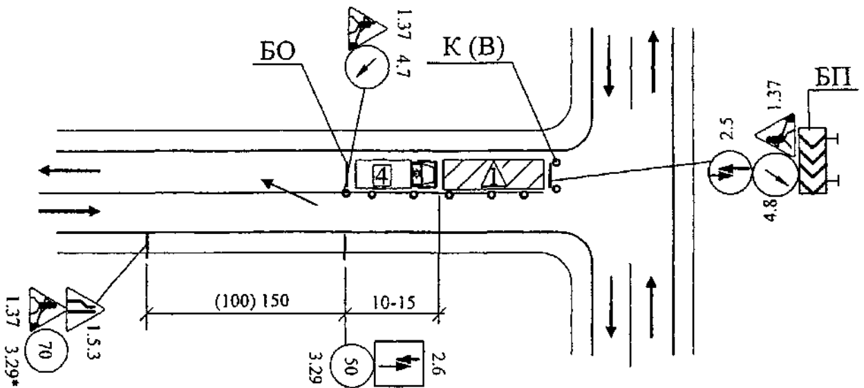
Схема А.13 Нанесення розмітки на примиканнях по трафаретах або лекалах ручною розмітною машиною
