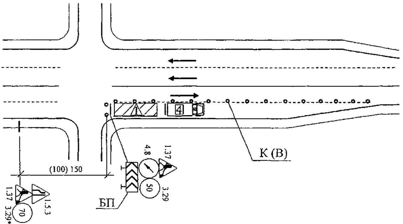
Схема А.12 Нанесення розмітки по трафаретах або лекалах на смузі розгону
