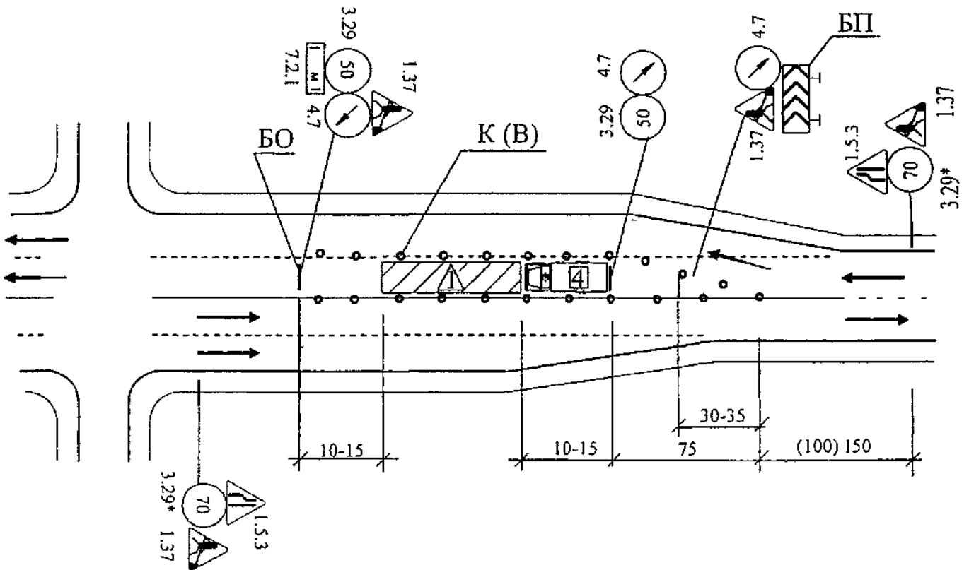
Схема А.10 Нанесення розмітки по трафаретах або лекалах на 2-х смугових дорогах з перехідно-швидкісною смугою
