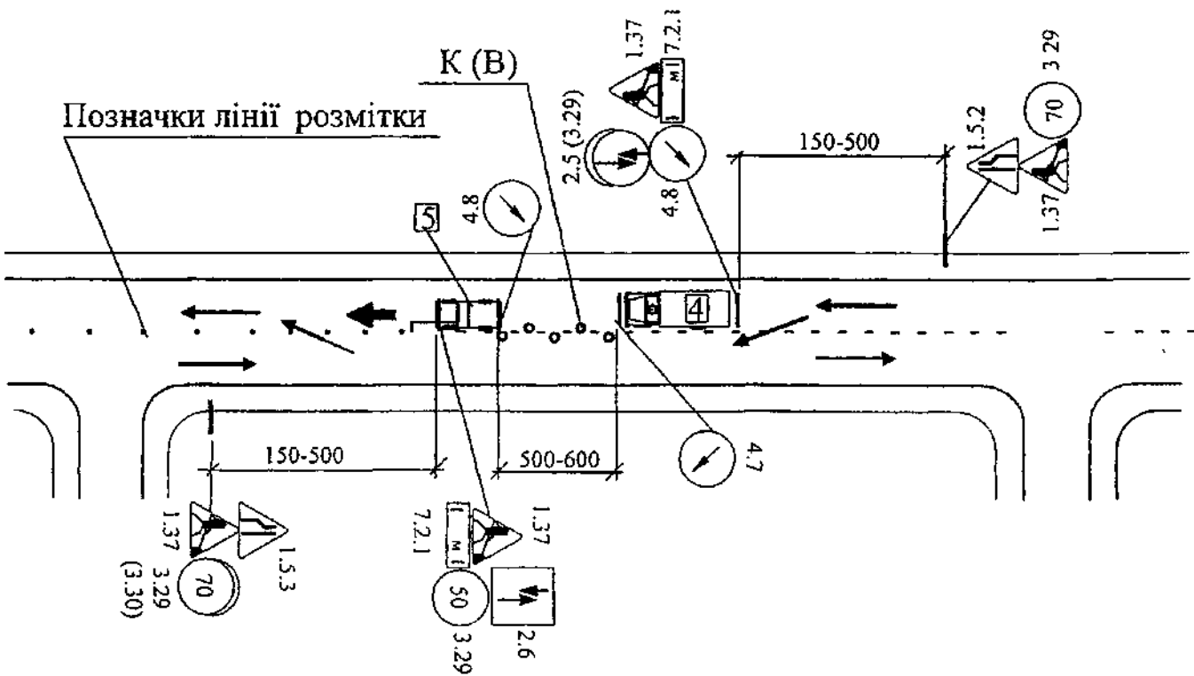
Схема А.6 Нанесення осьової лінії самохідною машиною
