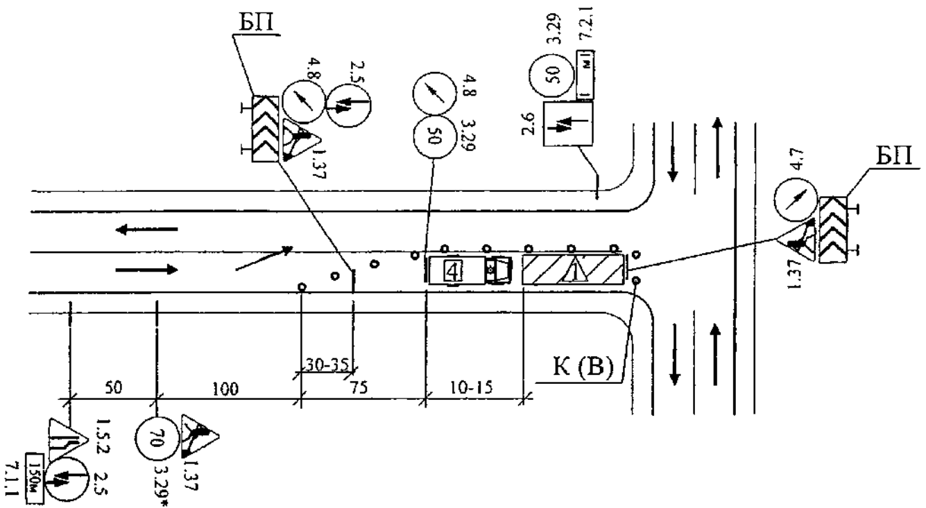
Схема А.13 Нанесення розмітки на примиканнях по трафаретах або лекалах ручною розмітною машиною
